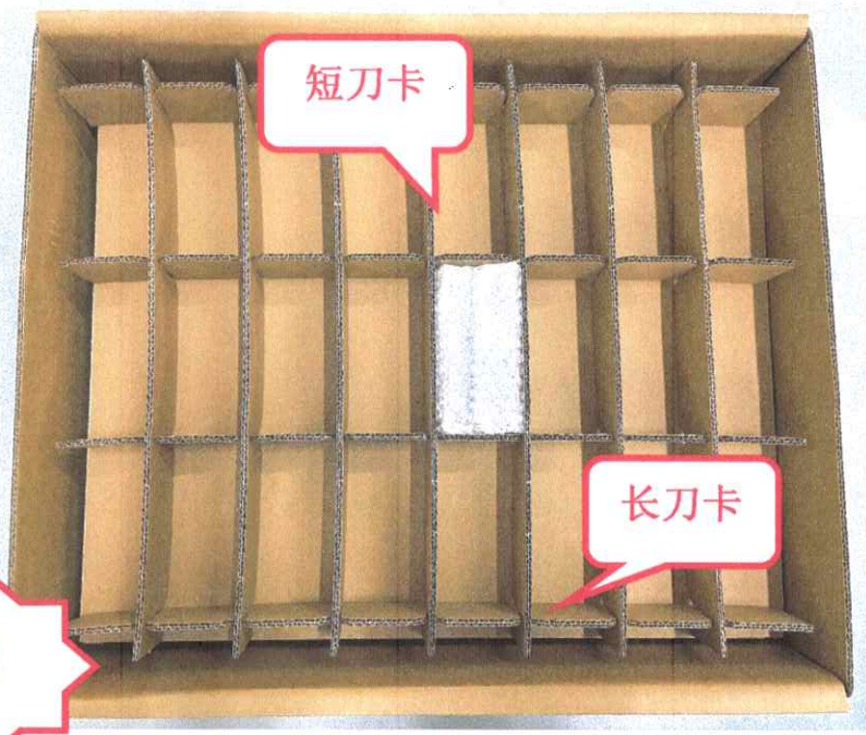
图三，每 1 个气泡袋装 5 个组件，每格放 4 袋 20 个，每层 24 格 480 个，每箱三层的方式包，共 1440 个，同时在底层，顶层各放 1 块隔板，中层 2 块。
